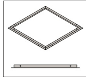
Inbyggingsram för montering i fast tak, se tillbehör. Skruvhålen i inbyggingsramen gör det möjligt att montera armaturen underifrån.
