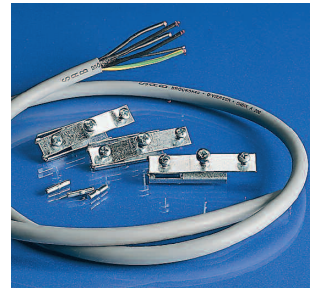
Överkopplingsats, för rampkoppling av armaturerna. Innehåller konfektionerad PVC-fri kabel 5x1,5 mm 2 samt dragstag och styrtift för hopkoppling av armaturerna - Ök sats 5307 för 28W. - Ök sats 5308 för 35W och 49W.
