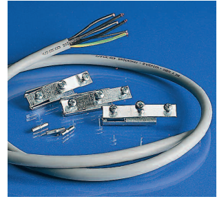
Överkopplingsats, för rampkoppling av armaturerna. Innehåller konfektionerad PVC-fri kabel 5x1,5 mm 2 samt dragstag och styrtstift för hopkoppling av armaturerna - Ök sats 5307 för 28W. - Ök sats 5308 för 35W och 49W.
