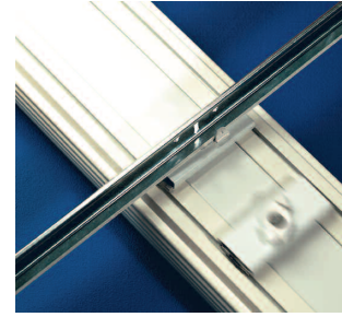
Som standard levereras armaturen med ställbara fästen för dikt montage mot T-profil (b=24 mm) kant A samt för fasta tak. Fästena är ställbara längs hela armaturen.
