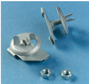
Vridclips 1839 , för kant A. Satsen innehåller 2 st wingmuttrar, 2 st M6 muttrar och 2 st vridklamrar.
