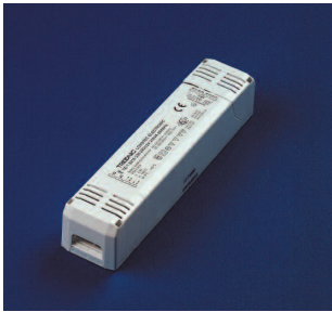
Elektronisk säkerhetstransformator med ljusreglering. Fabrikat Tridonic, TE one 4all (ljusreglering med switch DIM, DSI eller DALI) Klass II, IP20 Trafo 0402 , 105 VA, 230-240/12 V
