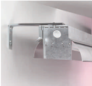
Armatur monterad på 90° konsol. Konsol 2013 , 90° (par).
