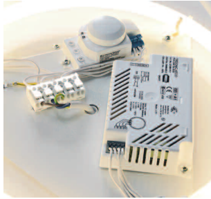
Varianterna med NS2, har sensorn monterad innanför kupan.
